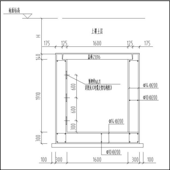
图 1.1-4 直线井土建断面图
