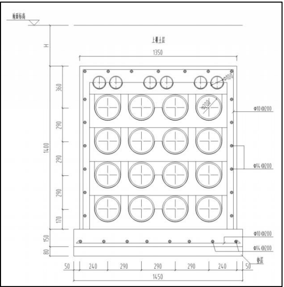
图 1.1-6 排管土建断面图
