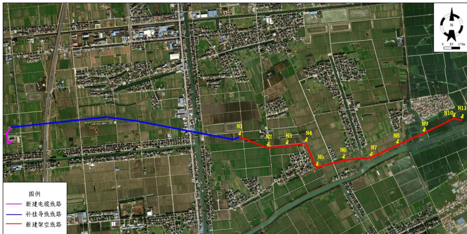
图 1.1-1 本工程线路路径走向图
