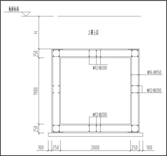
图 1.1-5 转角井土建断面图
