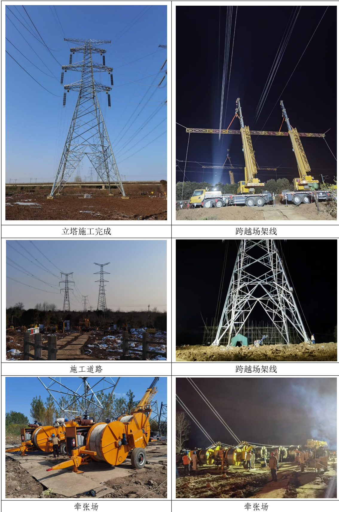
图 3-1 监测现场图
