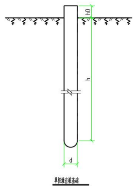
图 1.1-3 塔基基础示意图
