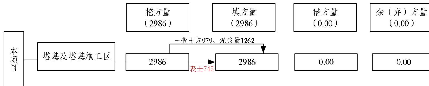
图 1.1-6 工程总土石方平衡流向框图 单位: m 3
