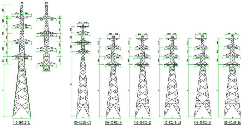
图 1.1-2 塔基型号图
