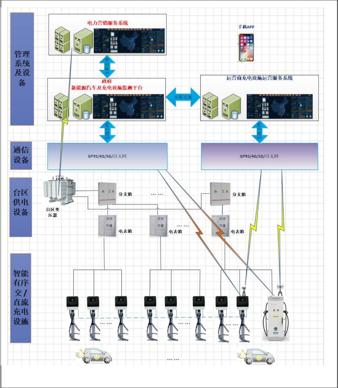
图1 有序充电系统架构
