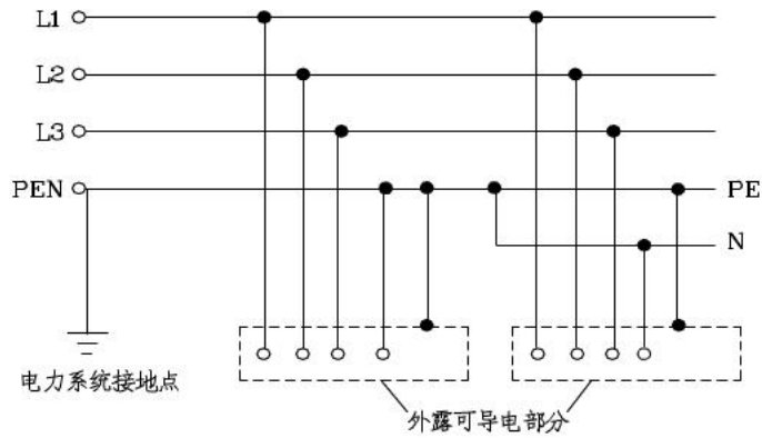
图 7.0.1-2 TN-C-S 系统
