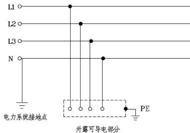
图 7.0.1-4 TT 系统
