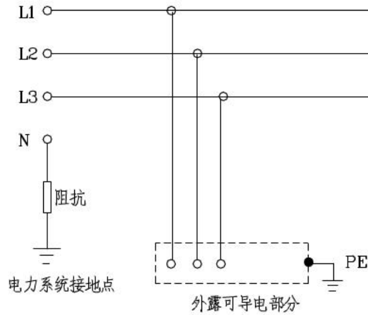
图 7.0.1-5 IT 系统
