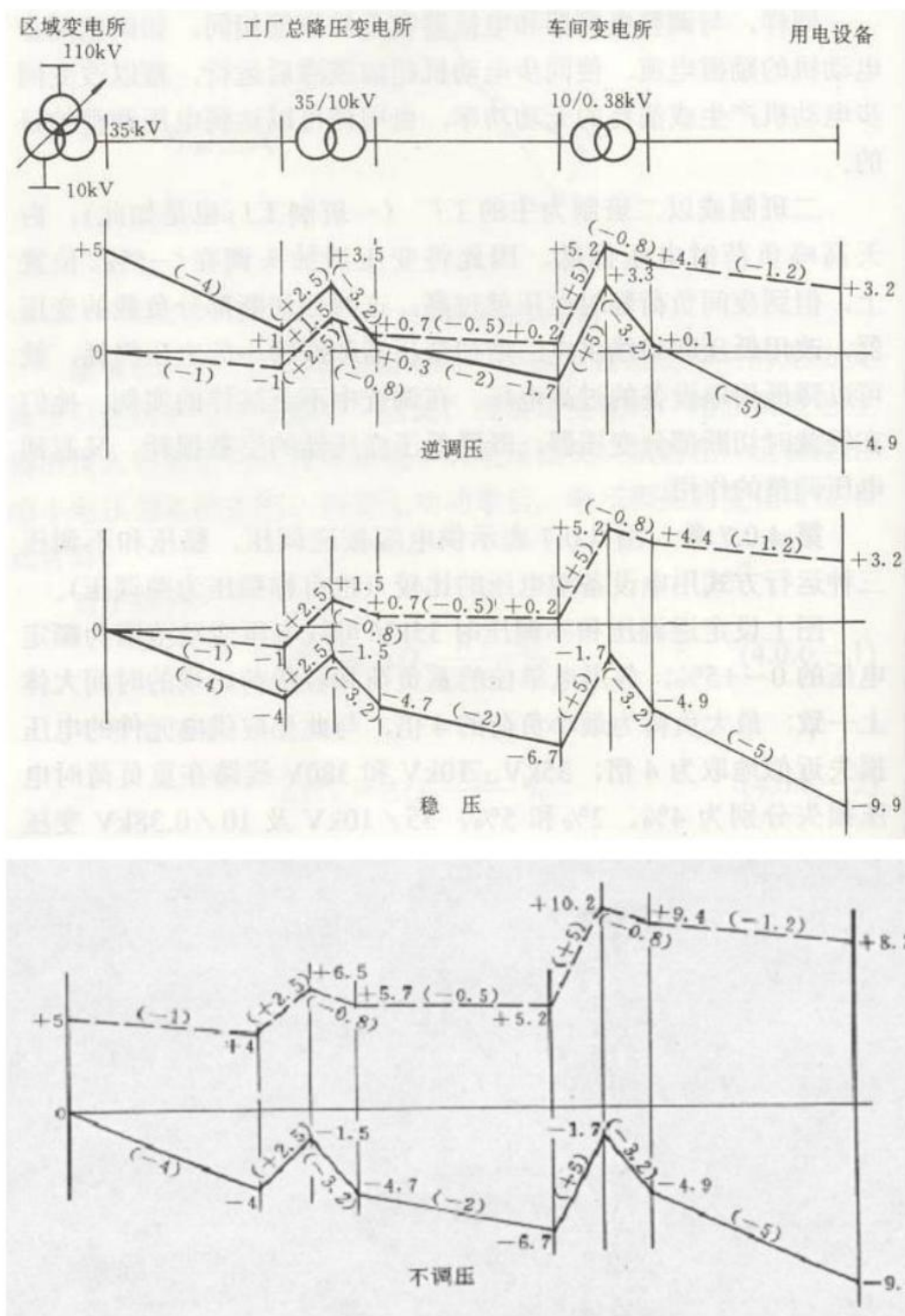
图 5.0.6 供电端按逆调压、稳压和不调压三种运行方式比较
