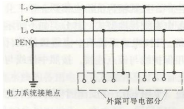
图 7.0.1-1 TN-C 系统
