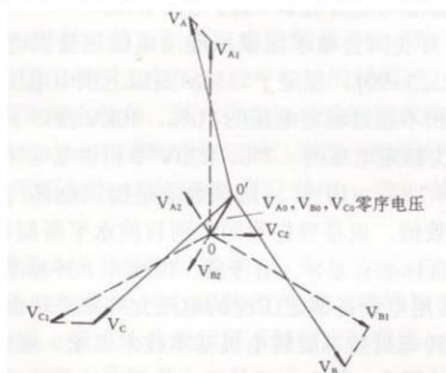
图 5.0.9 不对称电压向量图
