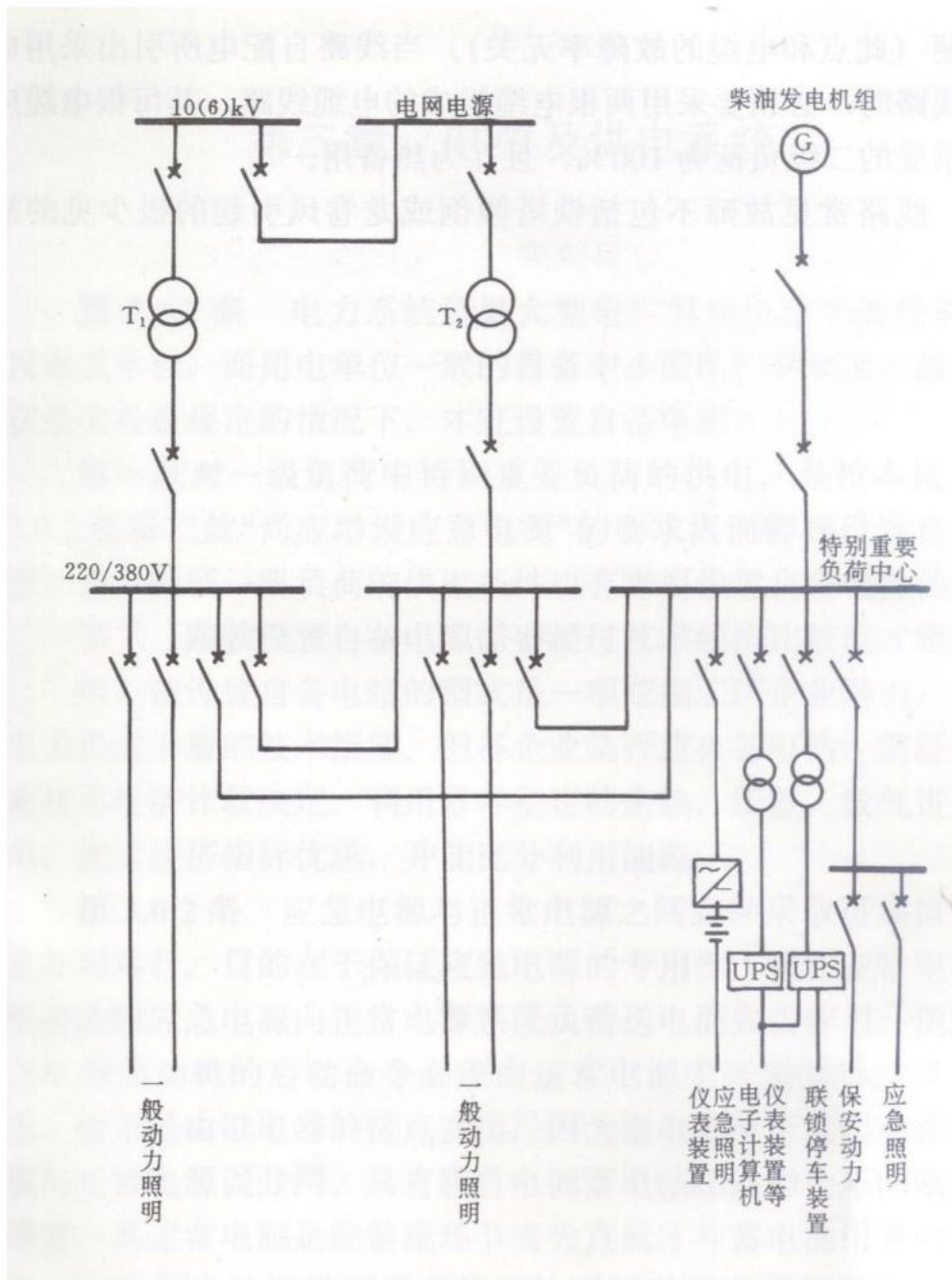
图 3.0.5 应急电源接线示例
