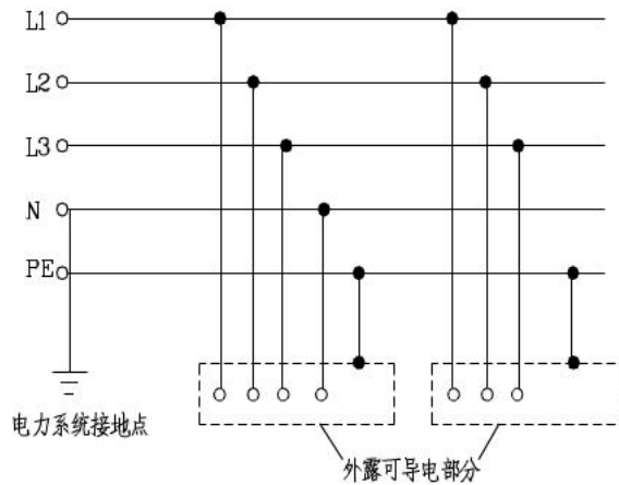
图 7.0.1-3 TN-S 系统
