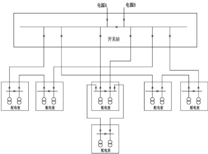
图 A.4 C 类供电方式
