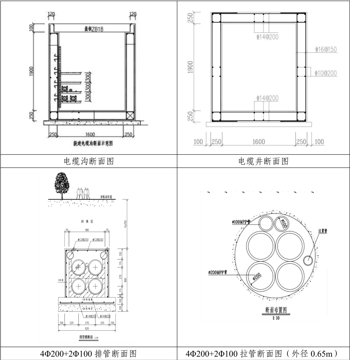
图 1.1-4 新建电缆断面图
