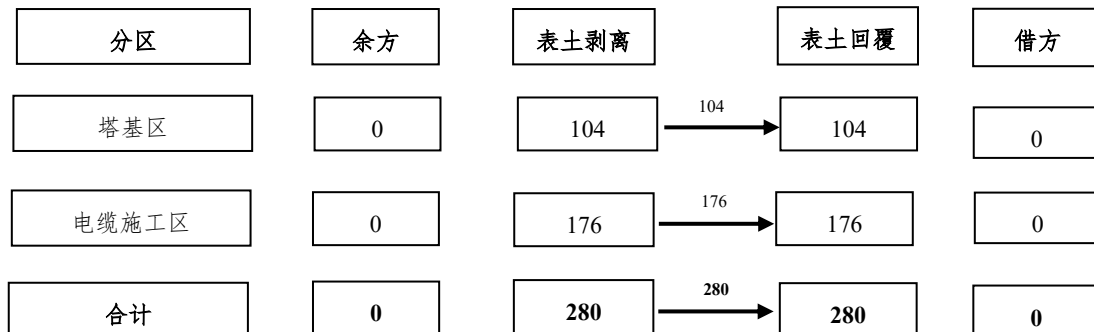
图 1.1-7 表土剥离平衡流向框图 单位: m 3
