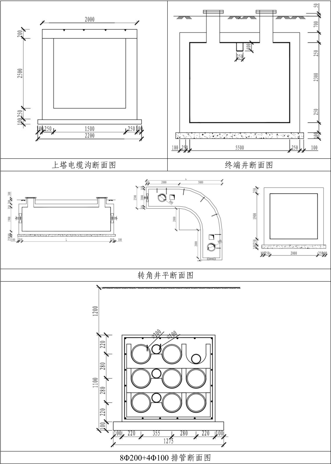
图 1.1-4 新建电缆断面图
