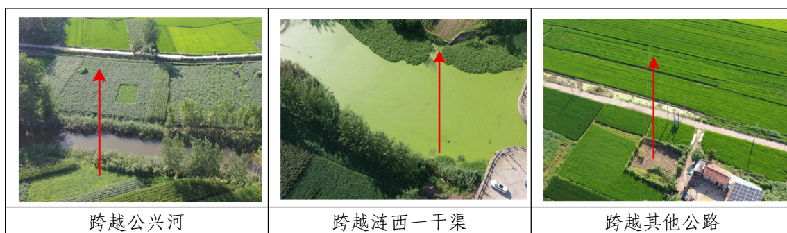
图 1.1-5 本工程架空线路跨越情况照片
