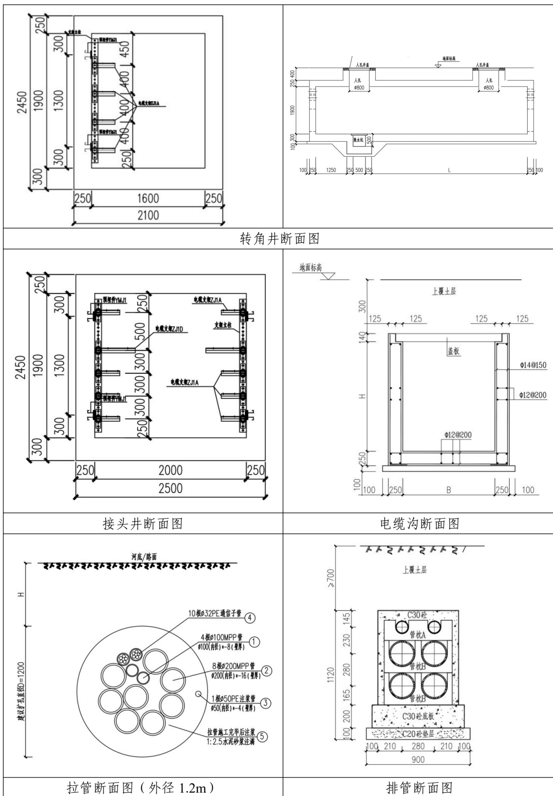
图 1.1-4 新建电缆断面图
